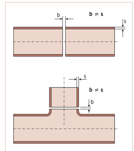
Stumpfnähte (I-Naht)
