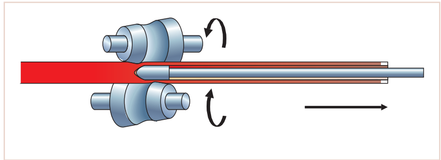
Warmsträgwalzen
