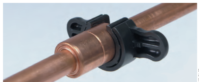
Beispiel für das nachträgliche Lösen einer Steckverbindung
