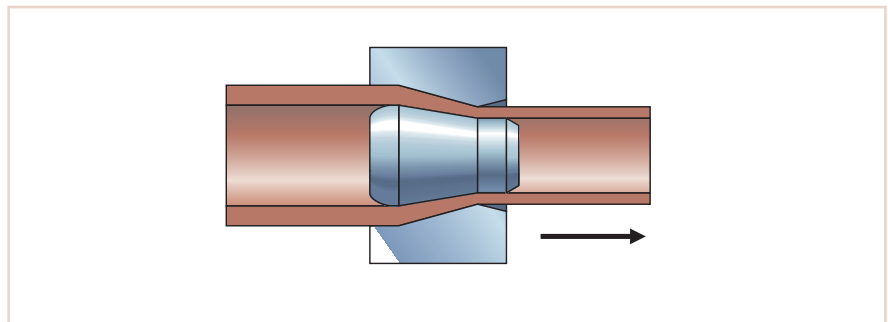
Kaltziehen mit fliegendem Dorn
