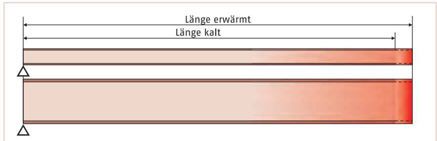
Die Längenänderung durch Wärmedehnung ist unabhängig vom Rohrdurchmesser
